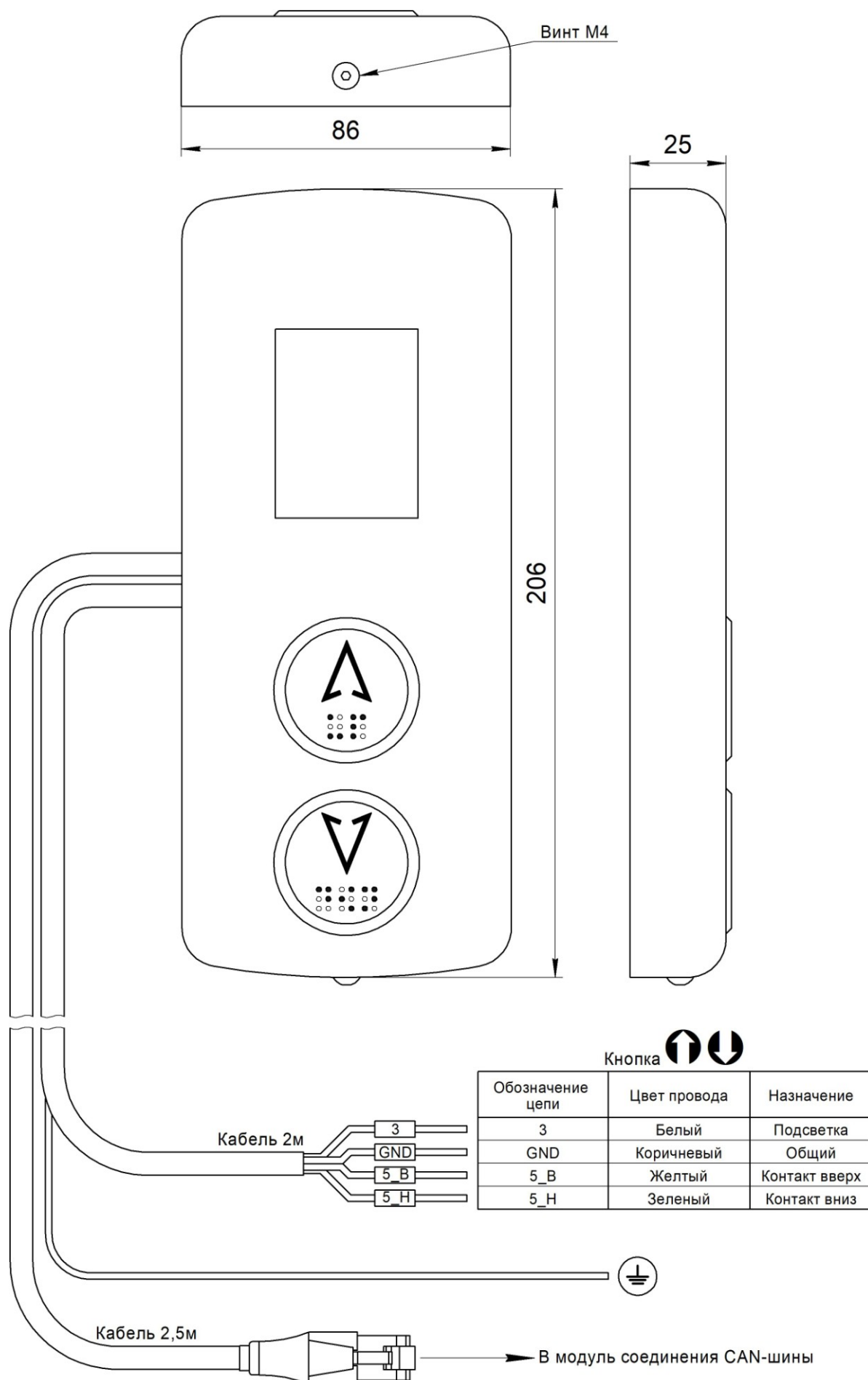
Рис.1 Внешний вид, габаритные и установочные размеры Вызывного поста ВП-2103-1086-08 (жгут RJ45)
